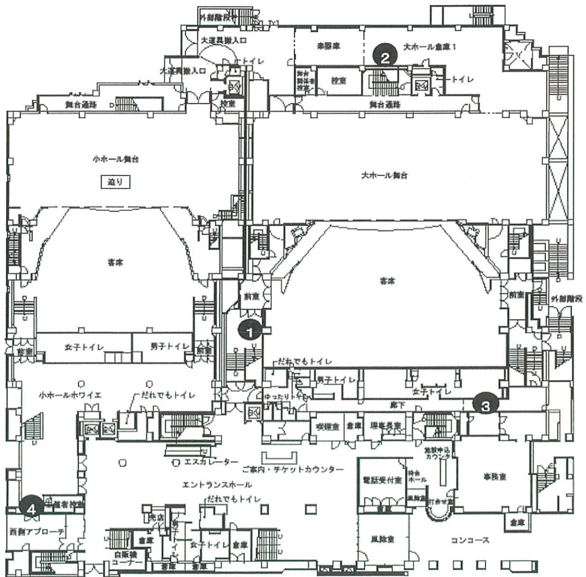
1階平面図
